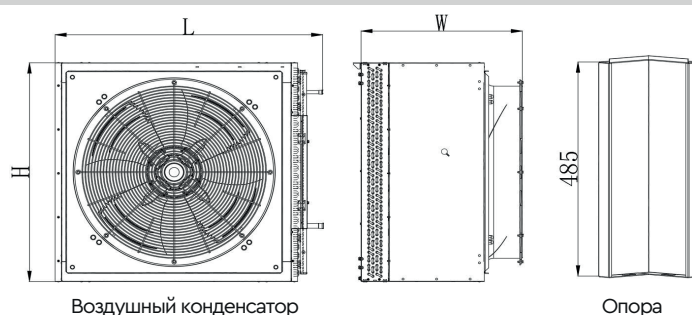
Воздушный конденсатор
