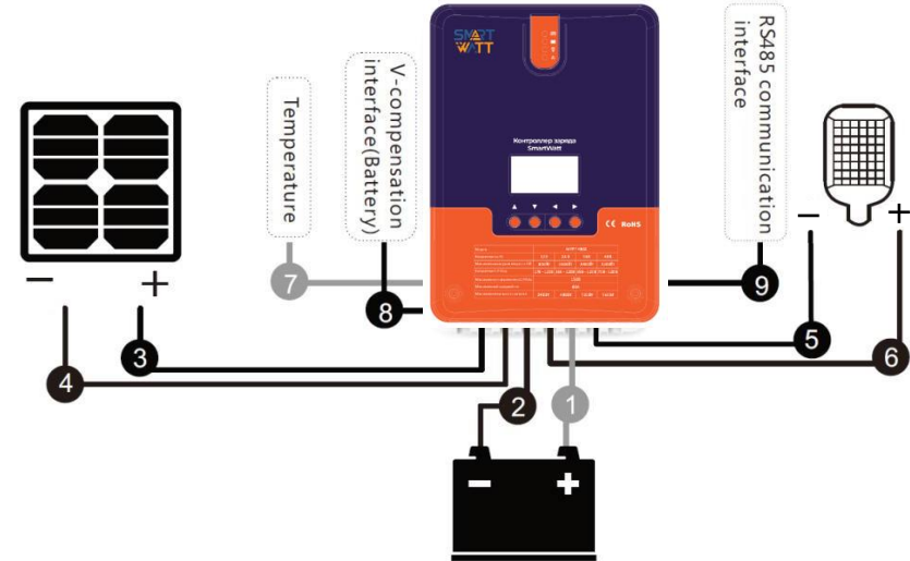
Рисунок 2-3. Последовательность монтажа проводов
