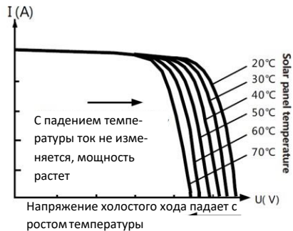
Рисунок 1-4. Зависимость выходных параметров модуля от температуры
