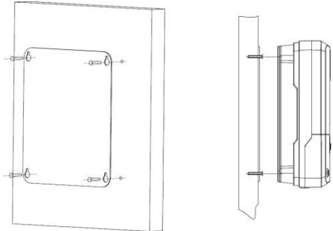
Рисунок 2.2. Последовательность монтажа
