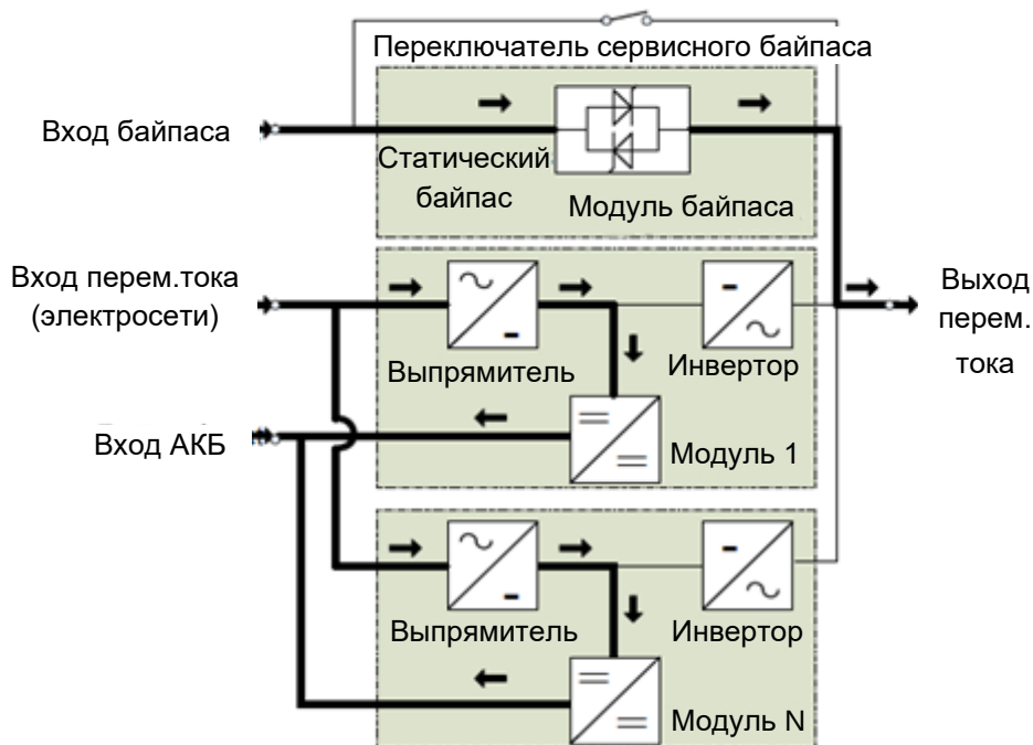
Рисунок 20. Схема работы ИБП в режиме байпаса.
