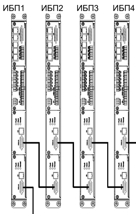
Рисунок 15. Параллельное подключение кабелей.
