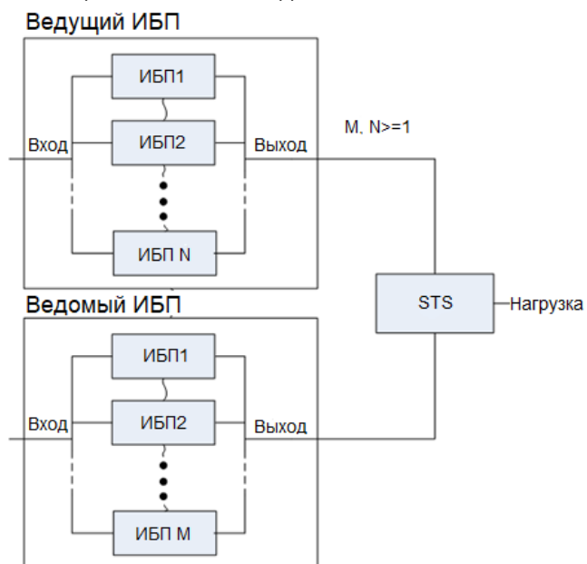
Рисунок 17. Общая схема всех подключенных систем.
