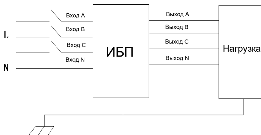
Рисунок 11. Общая схема подключения ИБП.
