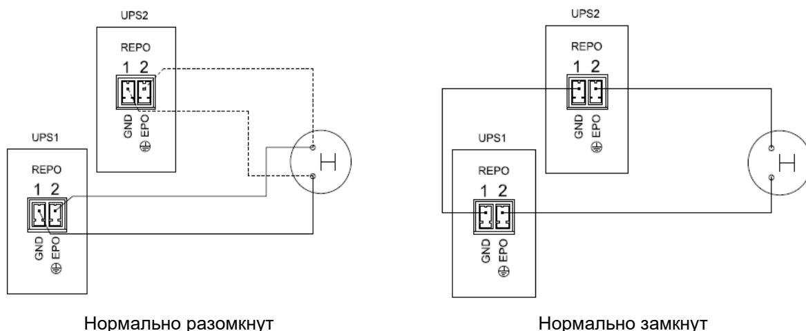
Рисунок 8. Внешний вид коммуникационного порта REPO.
