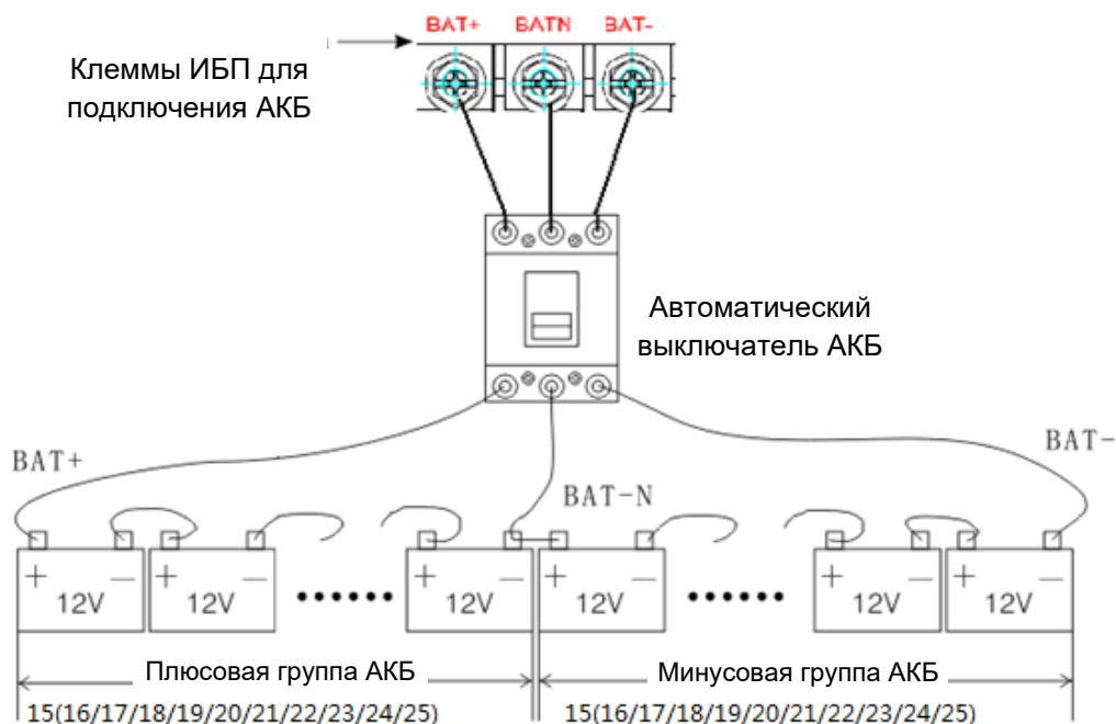
Рисунок 12. Схема подключения АКБ.
