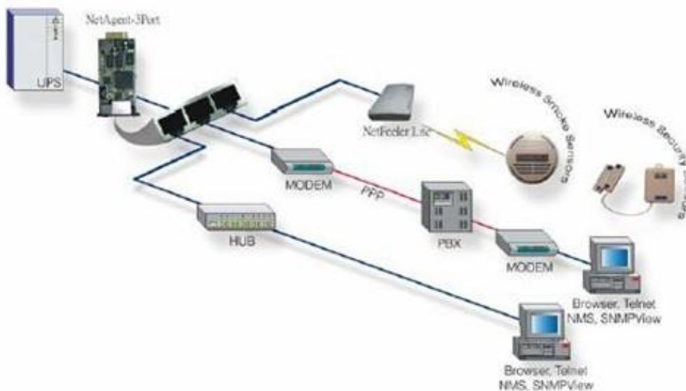
Рисунок 26. Стандартная топология сети управления ИБП.
