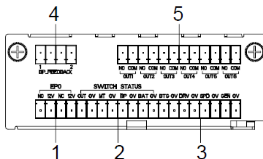
Рисунок 5. Внешний вид блока сухих контактов. Описание элементов см. в таблице Таблица .
