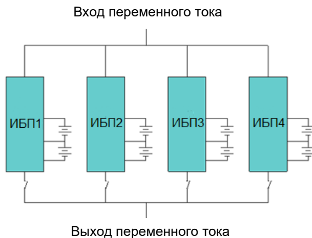
Рисунок 14. Общая схема параллельного соединения ИБП.
