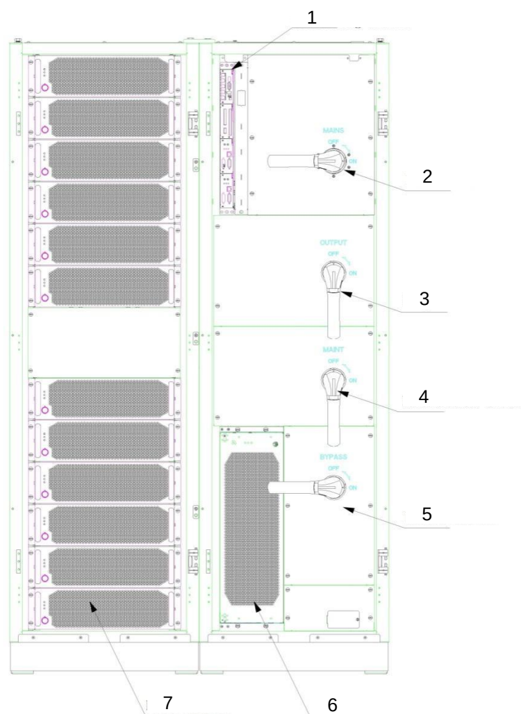
Рисунок 4. Вид изделия (400 – 600 кВт). Описание элементов представлено в таблице 2.
