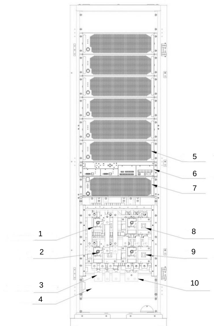
Рисунок 3. Вид изделия (200 – 300 кВт). Описание элементов представлено в таблице 1.
