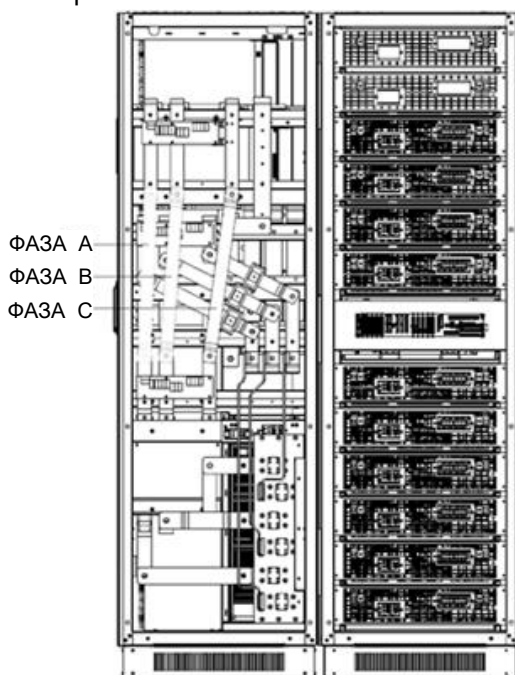
Рисунок 10. Фазы для подключения кабелей питания от сети переменного тока общего входа и байпаса.
