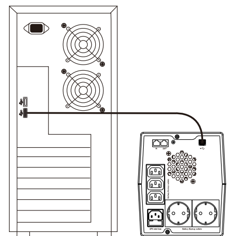
Рисунок 4. Подключение к компьютеру.
