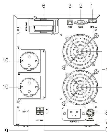
Рисунок 5. SMARTWATT UPS XPERT EURO 2kVA, вид сзади.
