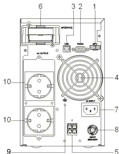
Рисунок 3. SMARTWATT UPS XPERT EURO 1kVA, вид сзади.
