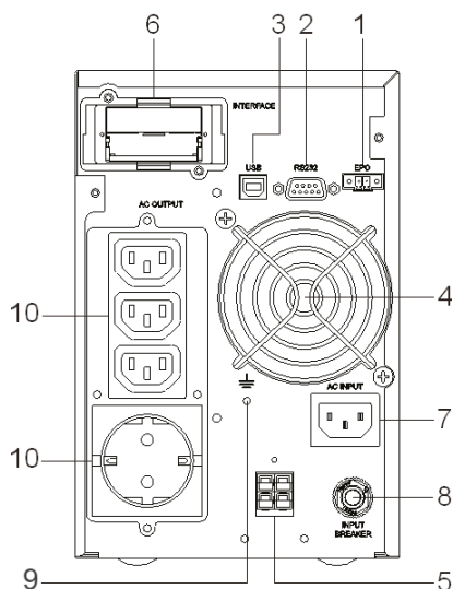
Рисунок 2. SMARTWATT UPS XPERT 1kVA, вид сзади.
