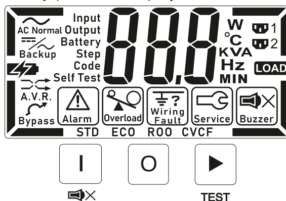
Рисунок 9. ЖК-дисплей и кнопки управления.
