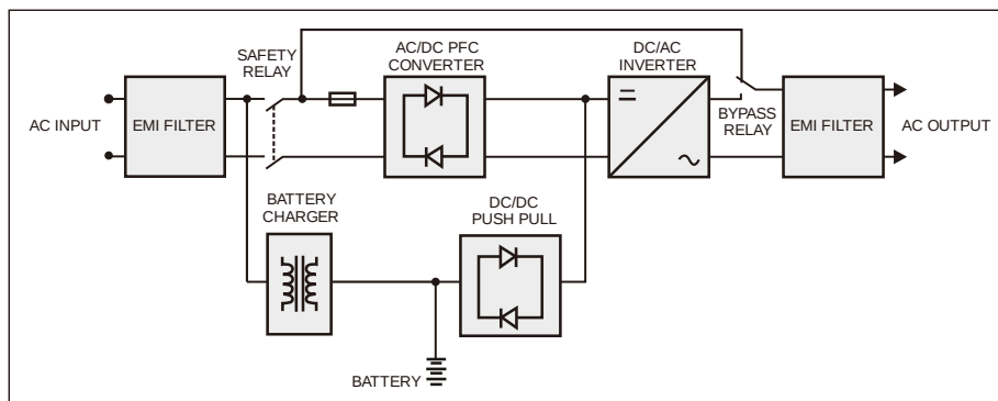
Рисунок 8. Блок-схема ИБП.
