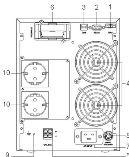
Рисунок 7. SMARTWATT UPS XPERT EURO 3kVA, вид сзади.
