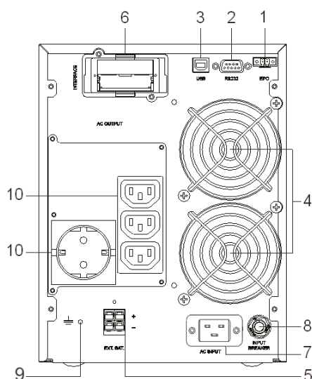
Рисунок 6. SMARTWATT UPS XPERT 3kVA, вид сзади.
