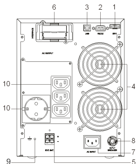
Рисунок 4. SMARTWATT UPS XPERT 2kVA, вид сзади.
