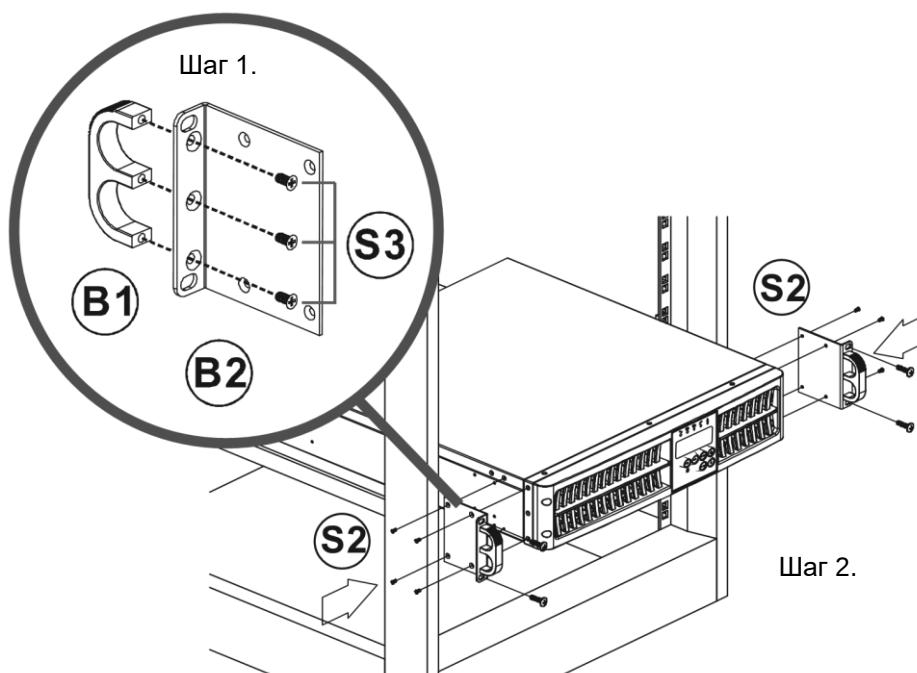
Рисунок 6. Установка кронштейнов для монтажа в стойку.
