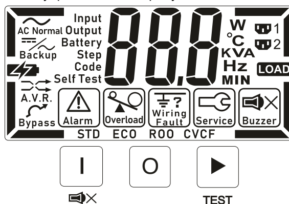
Рисунок 8. ЖК-дисплей и кнопки управления.
