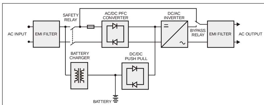
Рисунок 7. Блок-схема ИБП.
