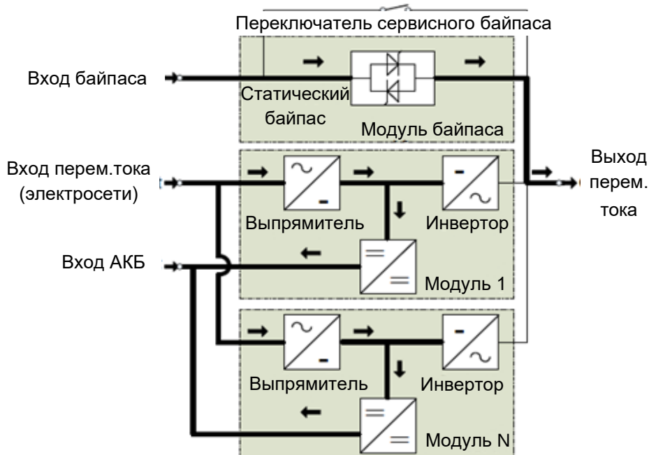
Рисунок 19. Схема работы ИБП в режиме ECO.
