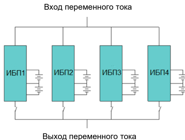
Рисунок 12. Общая схема параллельного соединения ИБП.
