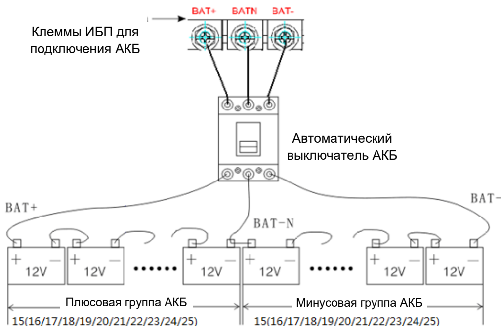
Рисунок 10. Схема подключения АКБ.
