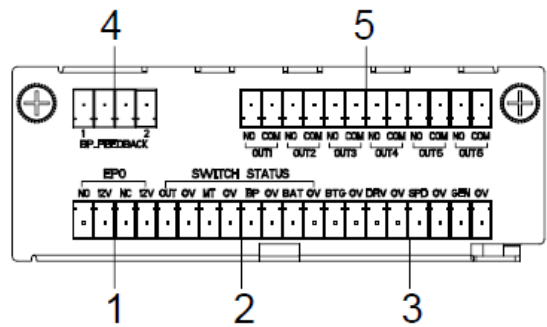
Рисунок 3. Внешний вид блока сухих контактов. Описание элементов см. в таблице Таблица .
