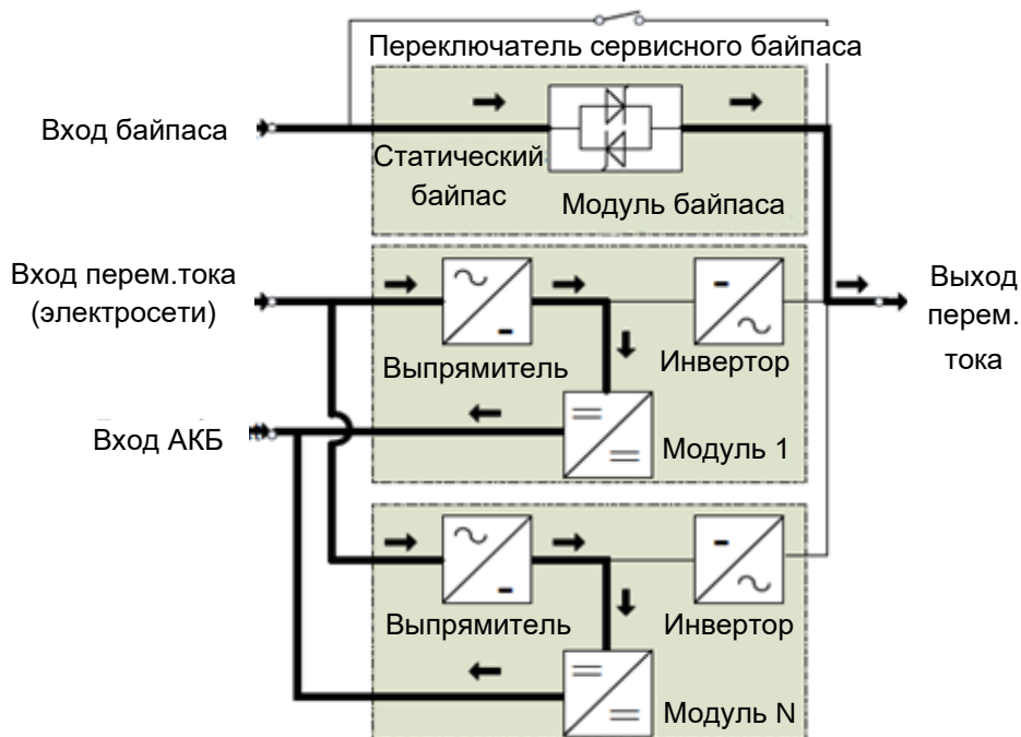
Рисунок 18. Схема работы ИБП в режиме байпаса.
