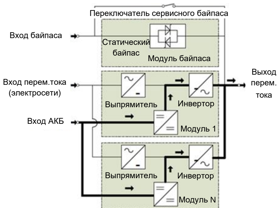
Рисунок 17. Схема работы ИБП в режиме от АКБ.
