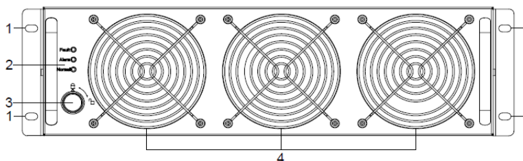
Рисунок 11. Модуль ИБП. Описание элементов см. в таблице 6.
