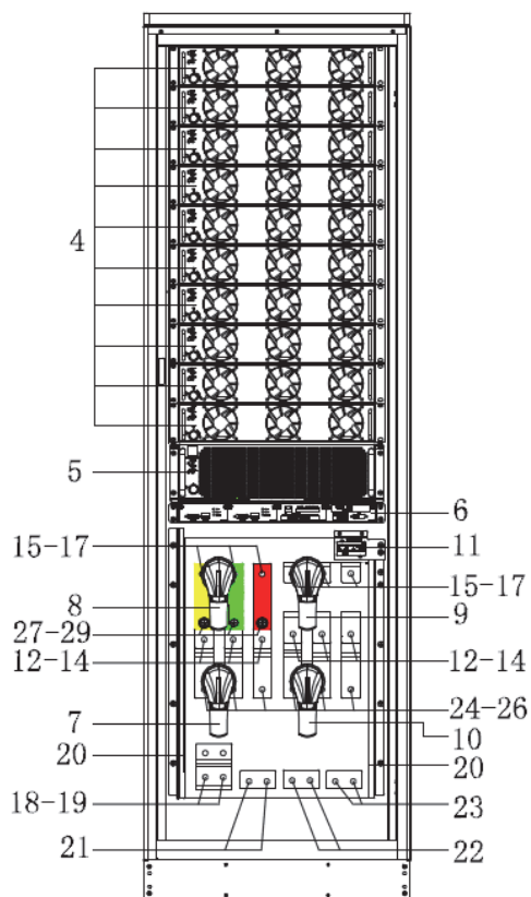
Рисунок 4. Вид изделия (200 – 300 кВА).
