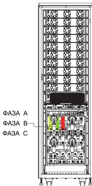
Рисунок 8. Фазы для подключения кабелей питания от сети переменного тока общего входа и байпаса.
