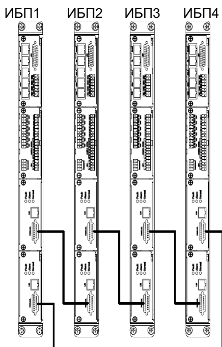
Рисунок 13. Параллельное подключение кабелей.
