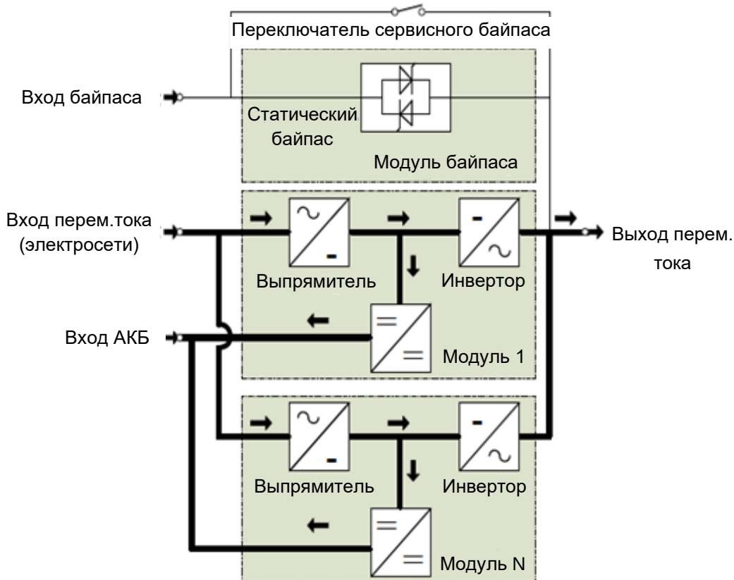
Рисунок 16. Схема работы ИБП в нормальном режиме.
