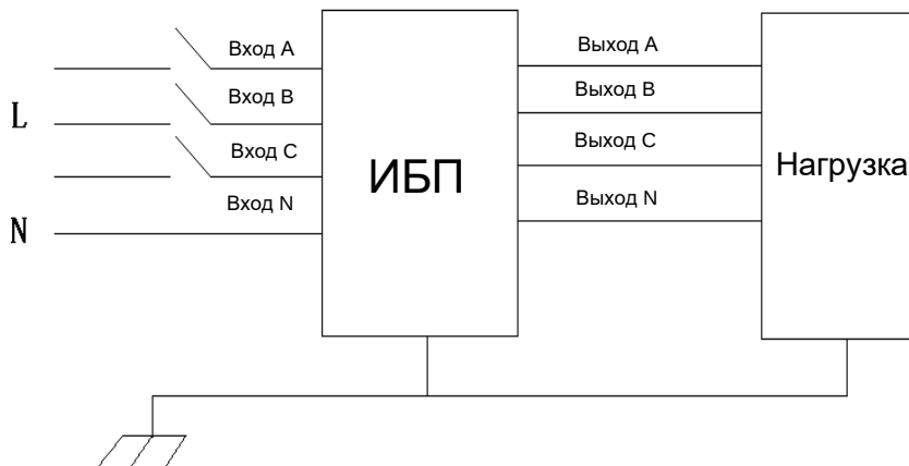
Рисунок 9. Общая схема подключения ИБП.
