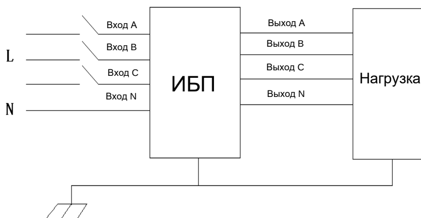
Рисунок 16. Общая схема подключения ИБП.
