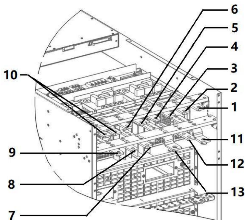
Рисунок 15. Фазы для подключения кабелей питания от сети переменного тока общего входа и байпаса.
