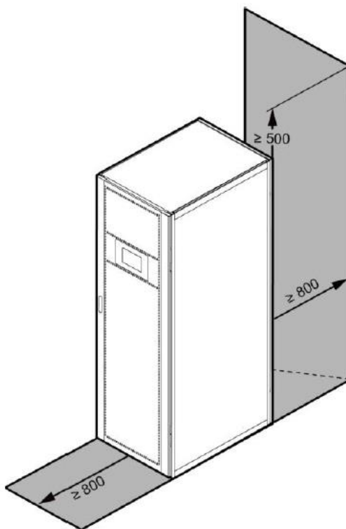
Рисунок 14. Требования к пространству для технического обслуживания.
