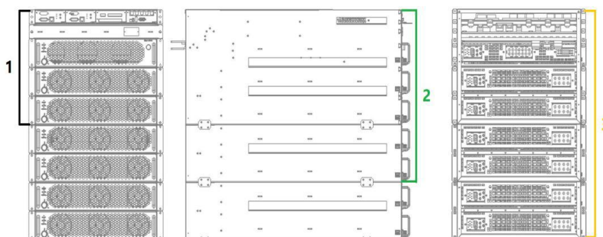
Рисунок 2. Внешний вид моделей (спереди/сбоку/сзади).
