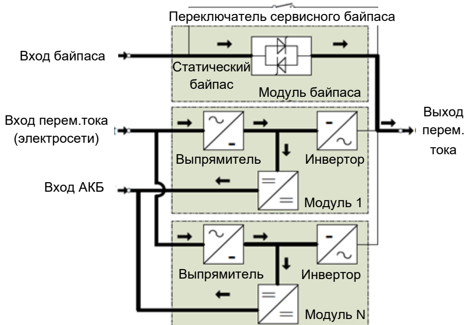
Рисунок 26. Схема работы ИБП в режиме ECO.
