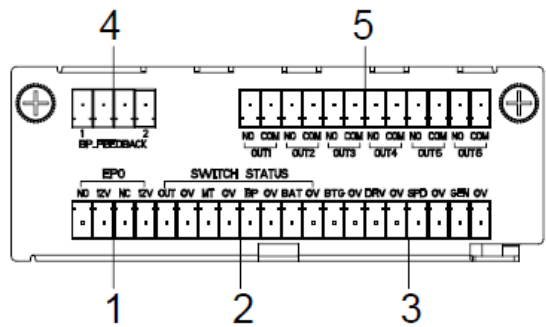
Рисунок 7. Внешний вид блока сухих контактов. Описание элементов см. в таблице Таблица .
