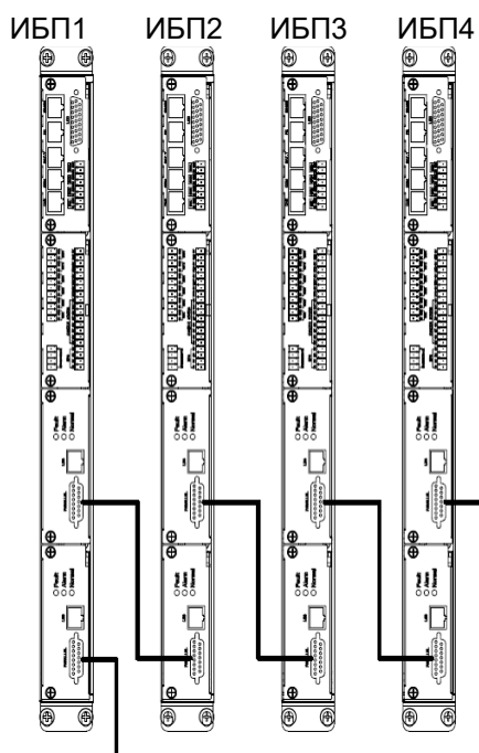
Рисунок 20. Параллельное подключение кабелей.
