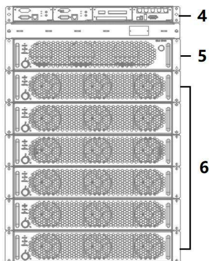
Рисунок 3. Вид шасси на 6 модулей (спереди).
