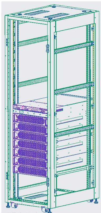
Рисунок 12. Установка шасси 19” телекоммуникационный шкаф
