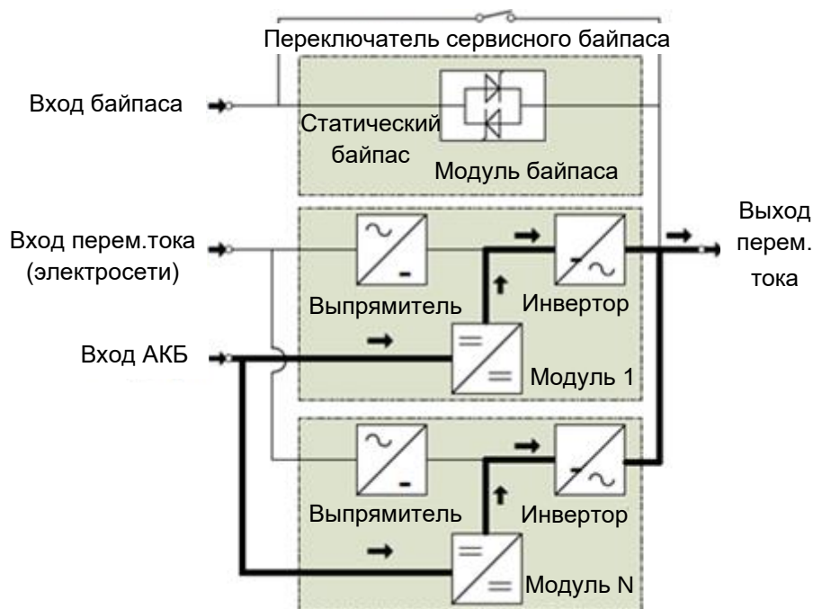
Рисунок 24. Схема работы ИБП в режиме от АКБ.
