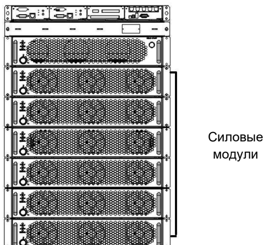
Рисунок 13. Шасси с установленными силовыми модулями (вид спереди)
