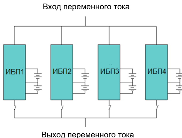
Рисунок 19. Общая схема параллельного соединения ИБП.
