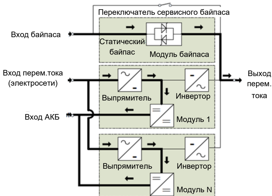
Рисунок 255. Схема работы ИБП в режиме байпаса.
