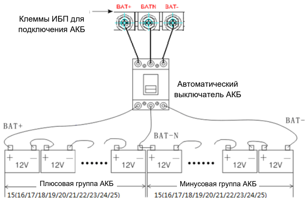
Рисунок 17. Схема подключения АКБ.
