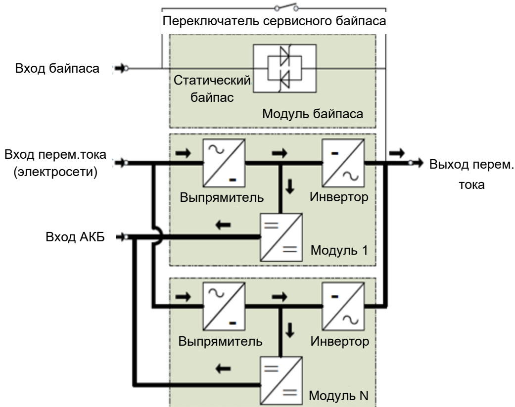
Рисунок 23. Схема работы ИБП в нормальном режиме.
