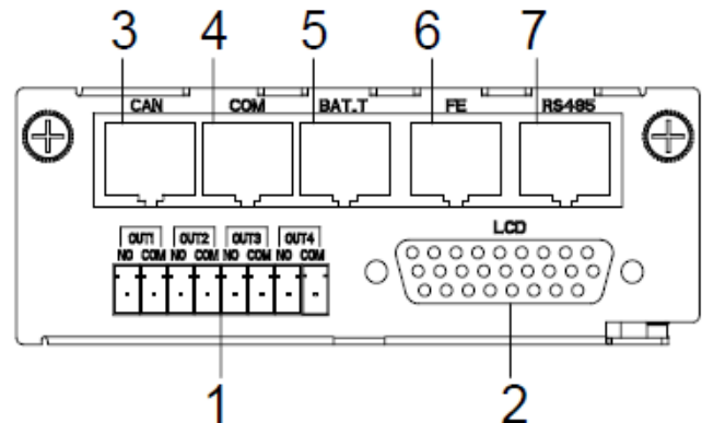
Рисунок 9. Внешний вид интерфейсного блока. Описание элементов см. в таблице Таблица .
