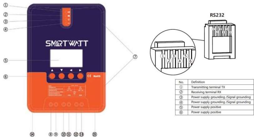
Рисунок 1. Внешний вид контроллера и распиновка разъема RS232.
