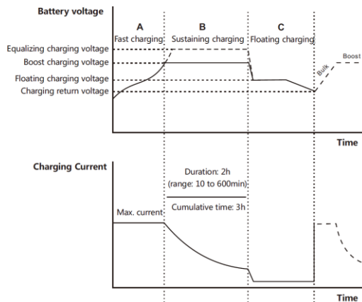
Рисунок 4. График этапов заряда аккумулятора
