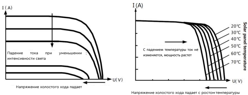
Рисунок 3. Зависимость выходных параметров панели от освещенности (слева) и температуры (справа)
