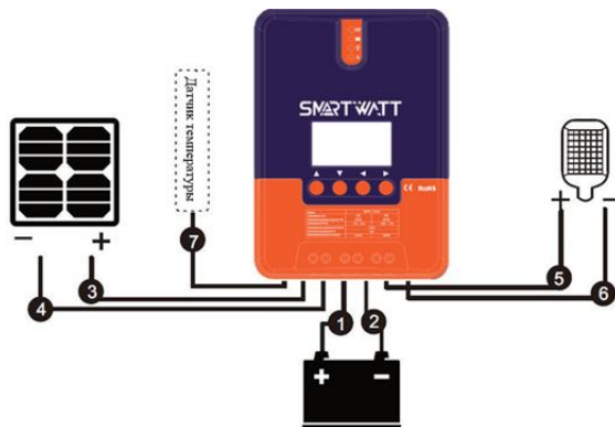
Рисунок 7. Схема подключения MPPT-контроллера
