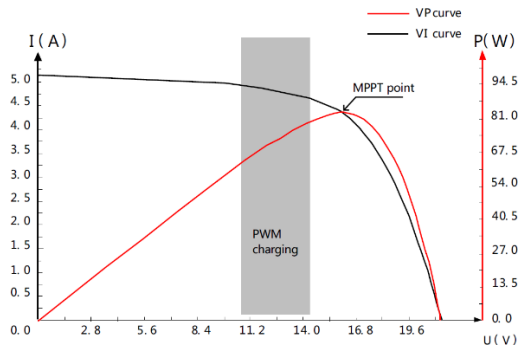
Рисунок 2. График выходных параметров солнечной панели
